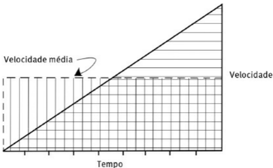
Gráfico da regra de Merton.
