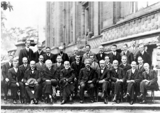
Pioneiros da teoria quântica na V Conferência Internacional de Solvay sobre Elétrons e Prótons, em Bruxelas, em 1927. Na última fila: Schrödinger (sexto a partir da esquerda), Pauli (oitavo), Heisenberg (nono). Na fila do meio: Dirac (quinto), Born (oitavo), Bohr (nono). Primeira fila: Planck (segundo), Einstein (quinto).
