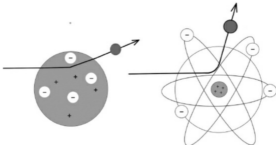
A prevista deflexão de partículas alfa nos átomos de Thomson (esquerda) e de Rutherford.
